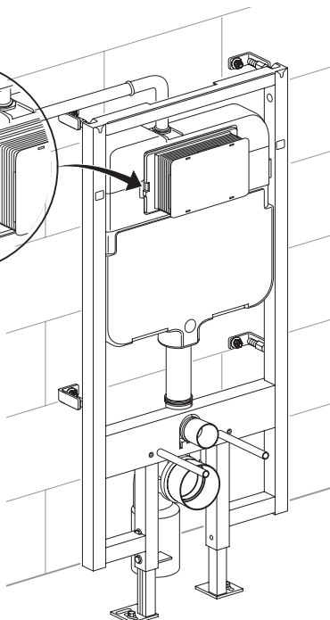
Phác họa lắp đặt khung kết nước
