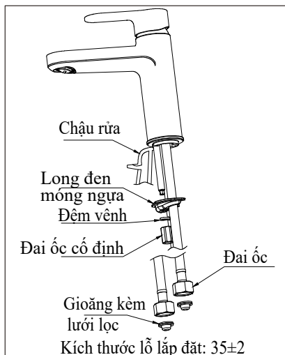
Hình 1: Lắp đặt thân vòi
