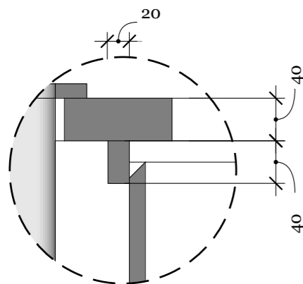
I Chi tiết cửa tủ 27-1 Tỷ lệ: 1:5
