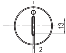
一字槽2X13mm型 Slot 2X13mm
