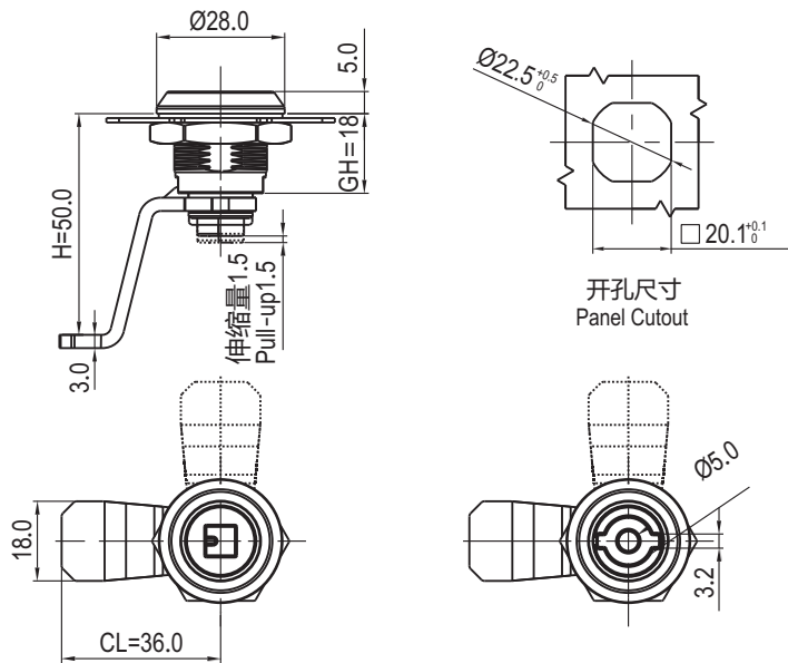
四方锁芯7 Square 7mm
