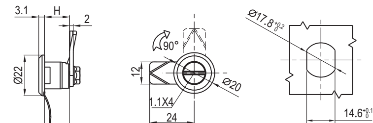
开孔尺寸 B Panel Cutout B
