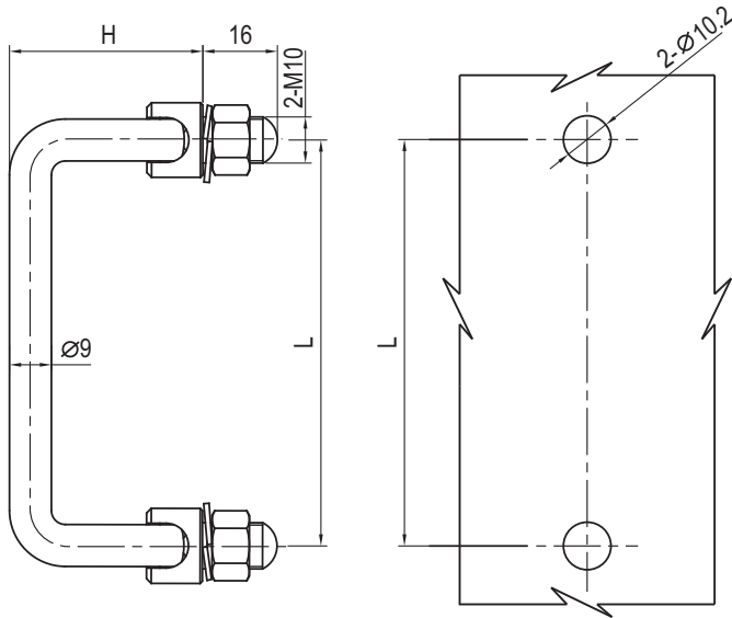
可折叠式拉手 Folding Handles
