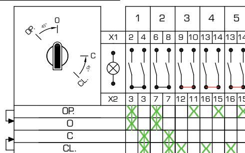
Circuit Arrangement n° DD5_15
