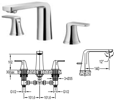
Vòi lavabo 3 món DVF-8236C-3 Giá: 8.600.000 VNĐ
