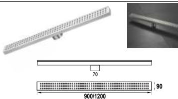
Xả sàn chống hôi dài 900mm DVQ-1014 Giá: 4.450.000 VNĐ 1200mm DVQ-1014-20 Giá: 6.450.000 VNĐ
