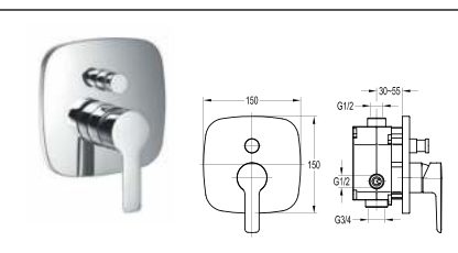
Khóa đóng mở 2 chức năng DVF-8308F-1 Giá: 5.150.000 VNĐ
