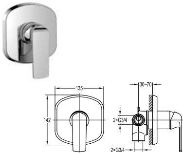
Khóa đóng mở 1 chức năng DVF-7309-1 Giá: 7.400.000 VNĐ
