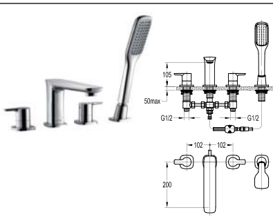
Vòi xả bồn 4 món DVF 9123 Giá: 12.200.000 VNĐ
