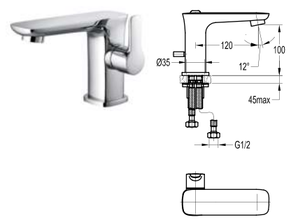
Vòi lavabo thấp DVF-9883-1 Giá: 6.200.000 VNĐ
