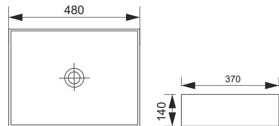
Lavabo đặt bàn màu đen DVQ-001-DB KT: 480*370*140mm Giá: 9.350.000 VNĐ
