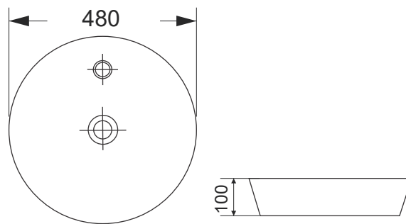
Lavabo đặt bàn RVT4386 KT: 480*480*100mm Giá: 2.990.000 VNĐ
