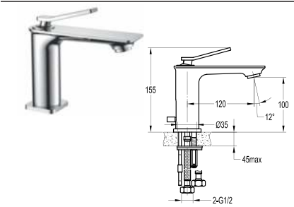
Vòi lavabo thấp DVF-9801-1 Giá: 4.750.000 VNĐ
