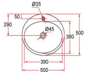
Lavabo đứng RVT49001 KT: 500*500*840mm Giá: 10.150.000 VNĐ
