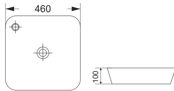
Lavabo đặt bàn RVT-4387 KT: 460*460*100mm Giá: 3.500.000 VNĐ
