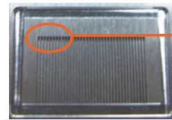
① 溝形状 Slot 溝幅：0.2mm Slot width 深さ：0.5mm Depth 長さ：5mm Length 溝数：36 本 Number of groove
