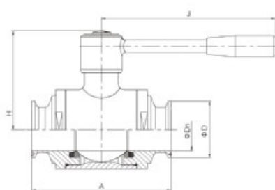
卡箍式 NO.VQC110S1
