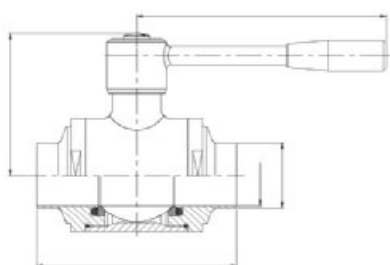
焊接式 NO.VQC100S1
