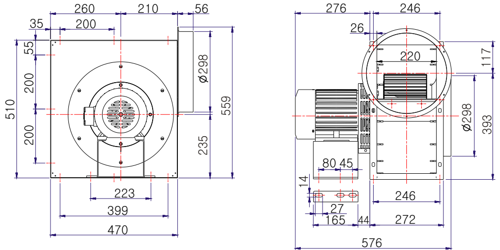
도면(Unit: mm)
