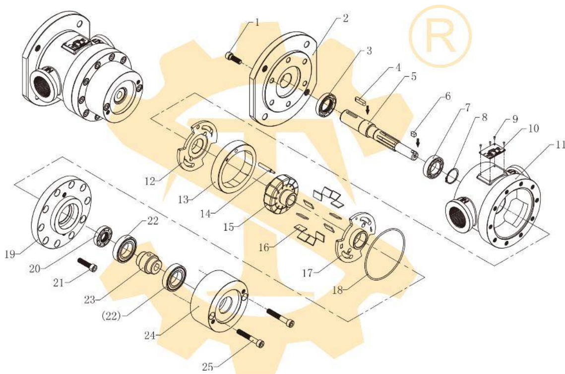
● 150T+B5-FR(LR) 零件表 / PARTS LIST
