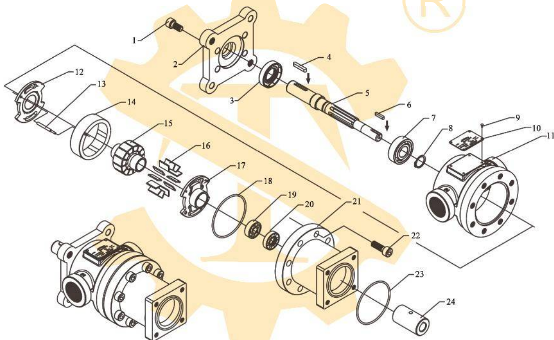
● 50T+PA-FR(LR)零件表 / PARTS LIST
