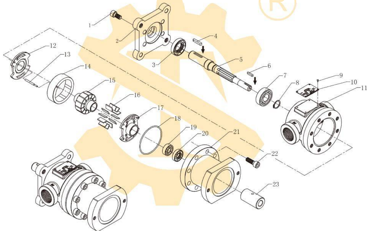
● 50T+B5-FR(LR) 零件表 / PARTS LIST
