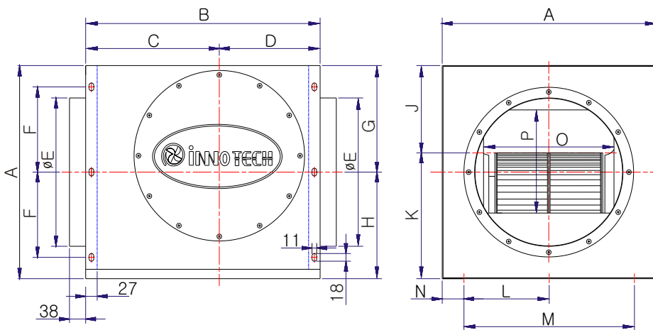
도면(Unit: mm)
