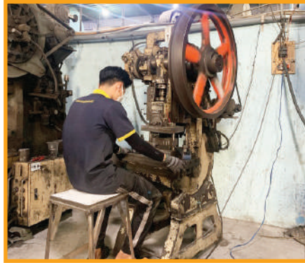
Máy đột dập cơ Mechanical punch press machine
