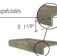
Elemento a L monolitico / HNT 3 16,5x30 6 1/2"x12" 075
