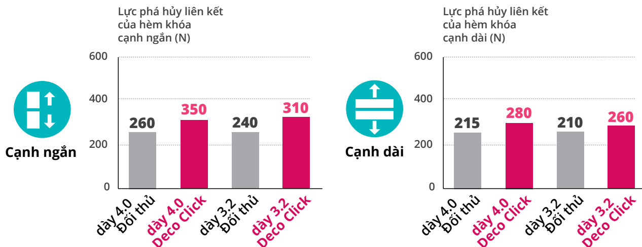
Bảng so sánh khả năng chịu lực hèm khóa
