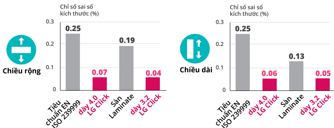
Bảng so sánh chỉ số sai số về kích thước
