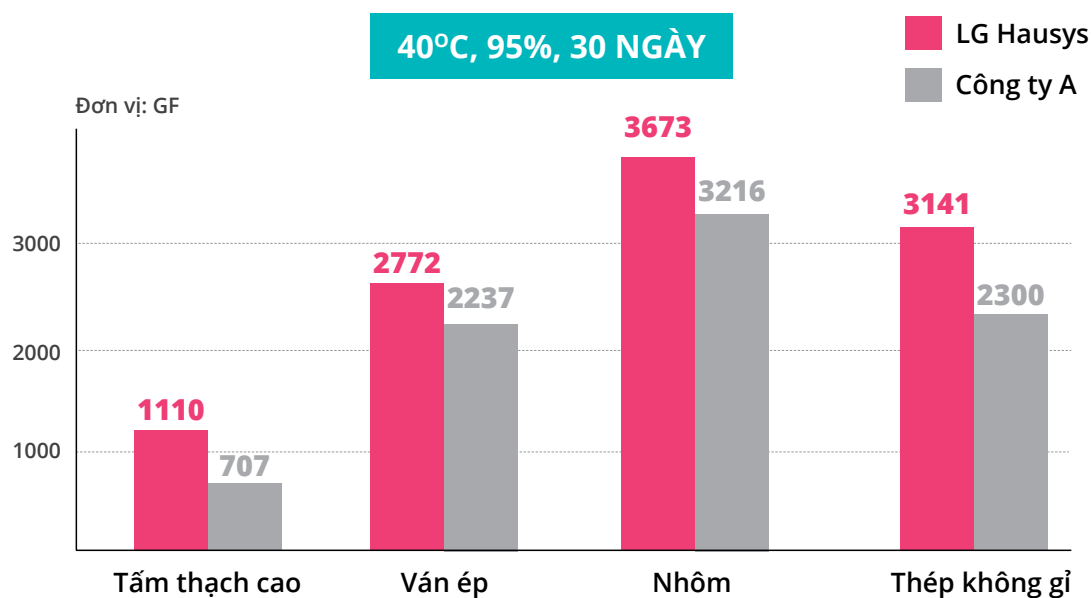
Bảng so sánh độ bám dính
